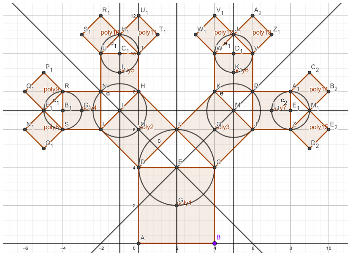
FIGURE 1 – Arbre de Pythagore avec 3 itérations réalisé dans Geogebra.
